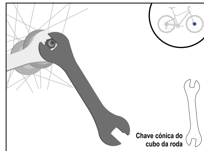
Ferramenta para disco de travão
