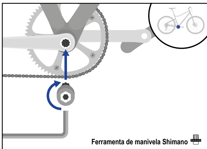
Chave de roda pedaleira
