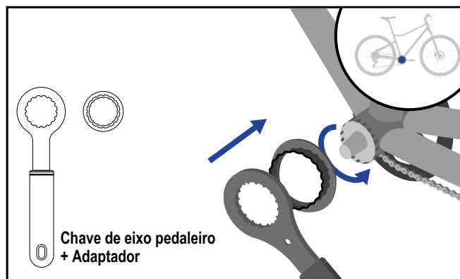
Extrator de manivela
