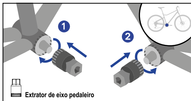
Chave de eixo pedaleiro + Adaptador
