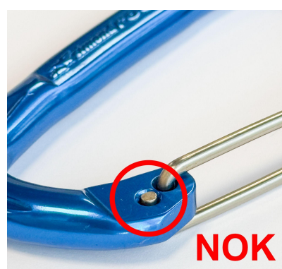
Foto 2: rebite NOK com extremidade plana
